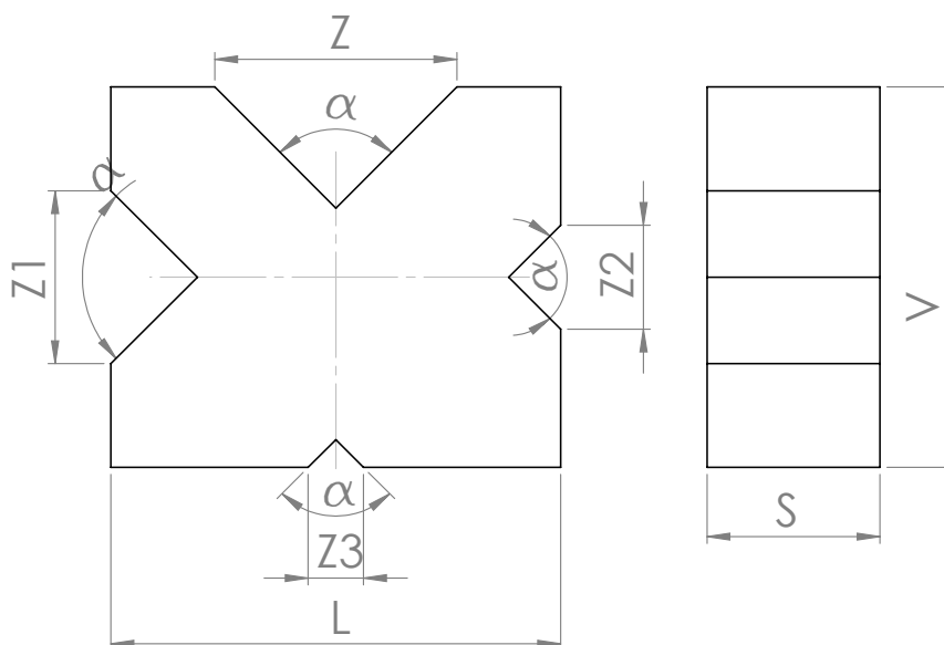
Kontrolní a rýsovací podložky se čtyřmi zářezy - pár
